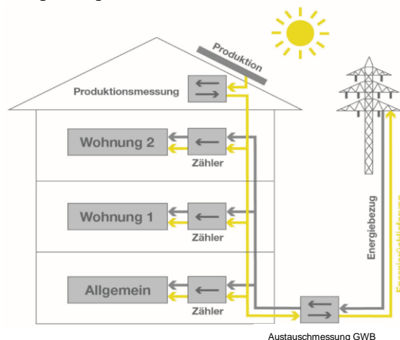
Abbildung 1: Messgeräteanordnung 1
