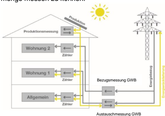
Abbildung 2: Messgeräteanordnung 2
